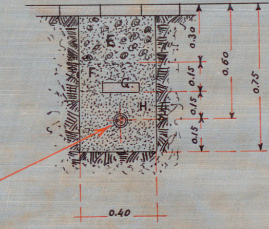
CORTE C.D.
