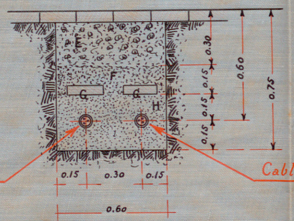
CORTE A.B.
